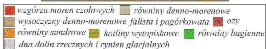
Rycina 4. Teren mpzp na tle fragmentu Przeglądowej Mapy Geomorfologicznej Polski. Źródło: Przyroda Pomorza Zachodniego, praca zbiorowa, Szczecin 2002 r.
