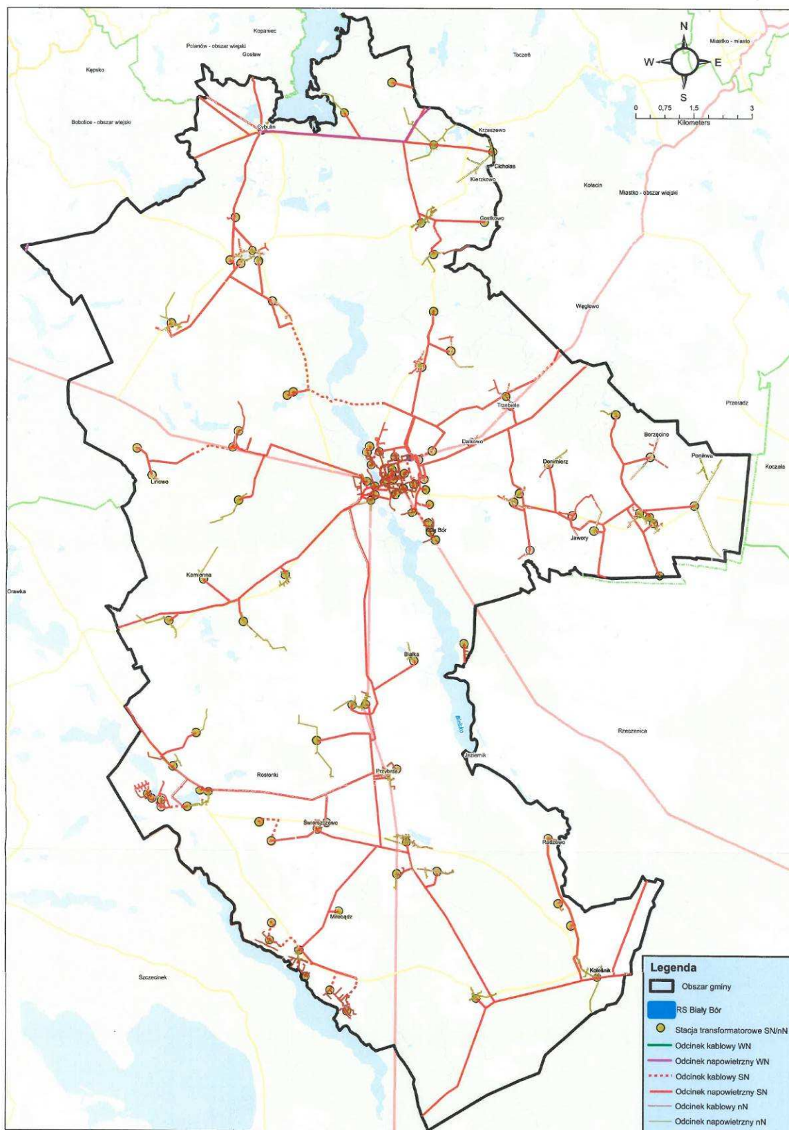
Rys. 18. Sieć elektroenergetyczna na obszarze miasta i gminy Biały Bór źródło: ENERGA -OPERATOR S.A. Oddział w Koszalinie
