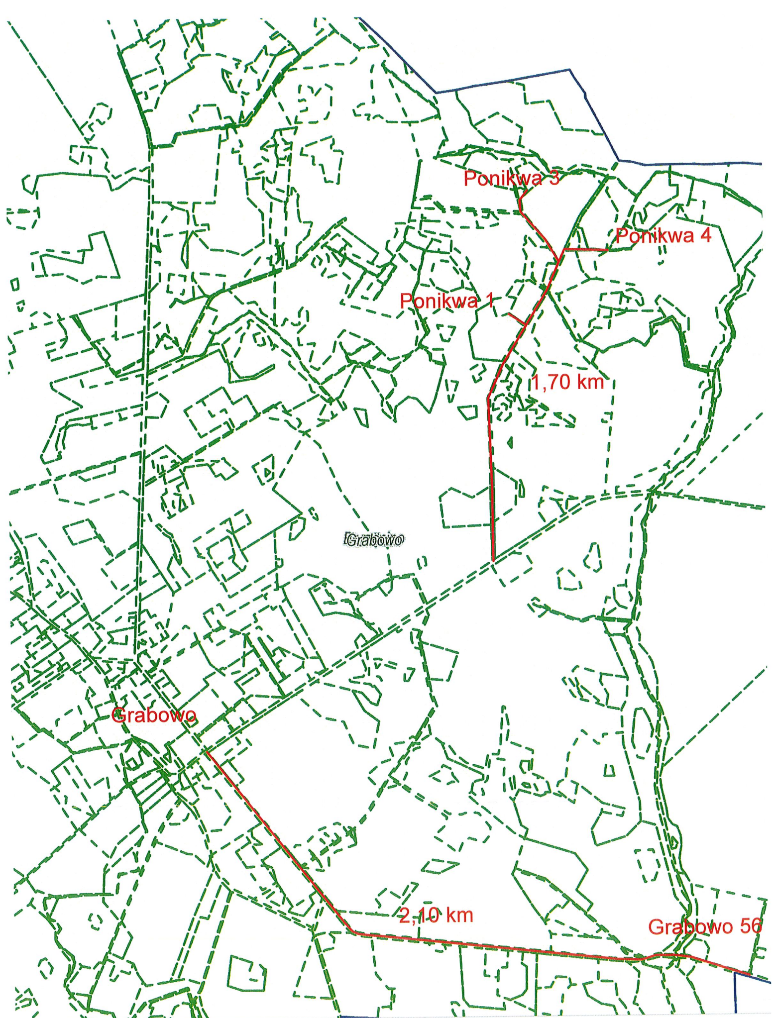
Rys. nr 8 - Grabowo-Pieniężnica, Ponikwa — zakres odśnieżania
