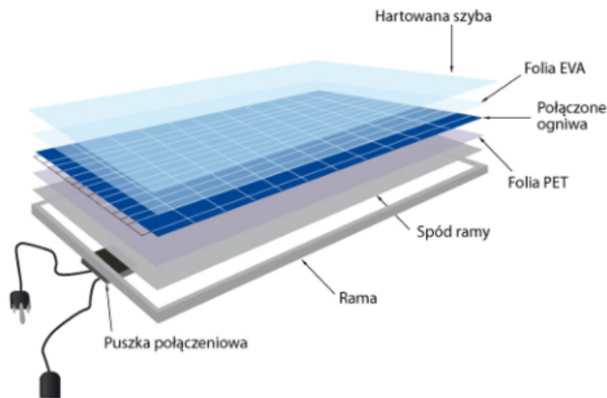
Rys. 3.2. Budowa panelu fotowoltaicznego
